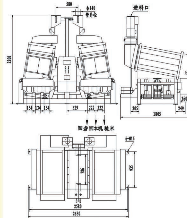
(外形尺寸与地脚安装图)
